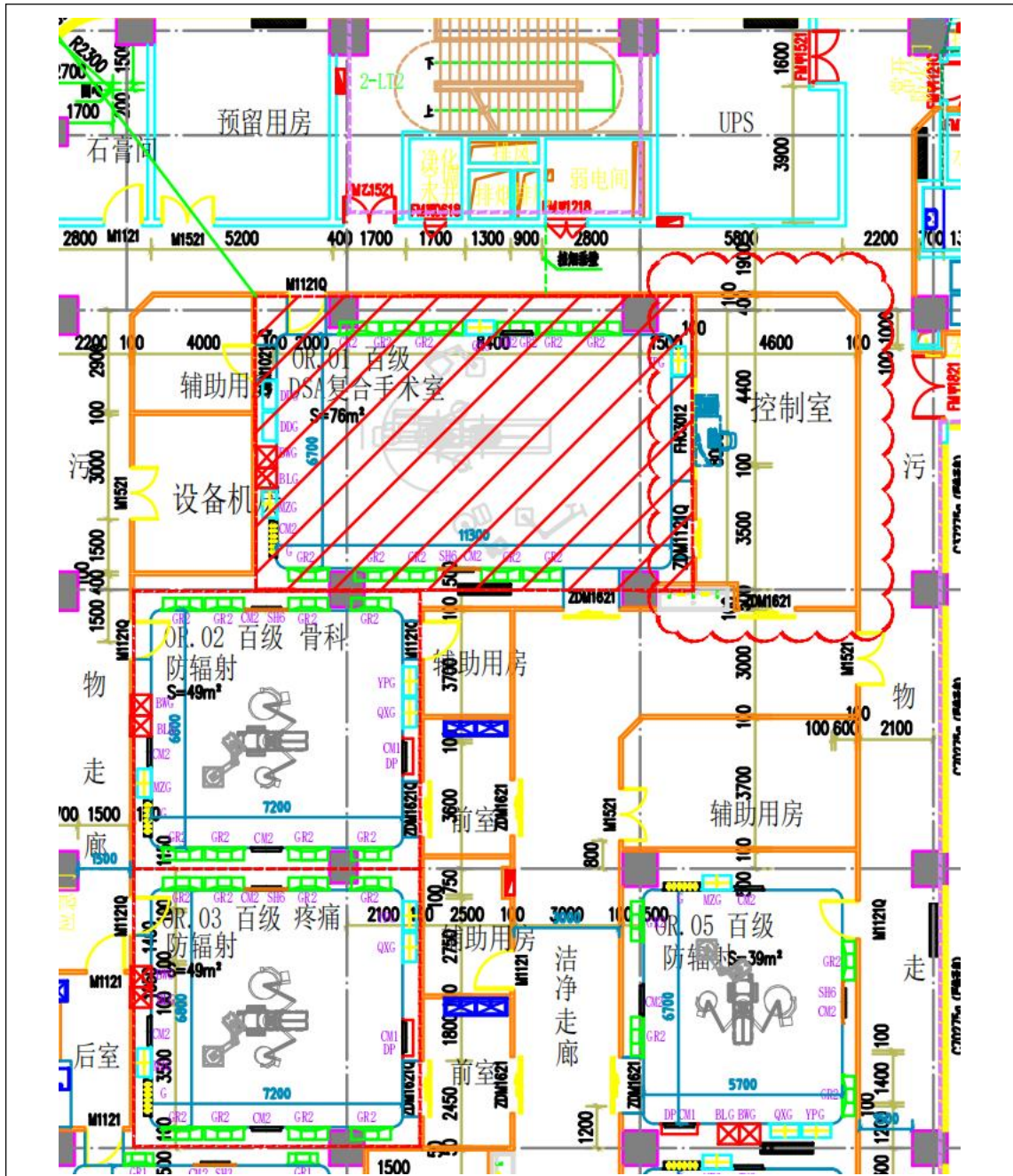
图 2-3 医技楼四楼手术中心 DSA 复合手术室
