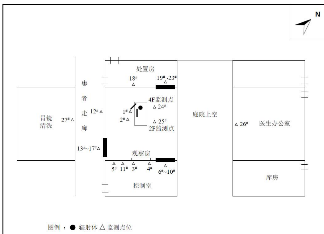
图 6-1 医技楼三楼 ERCP 室辐射环境监测布点示意图
