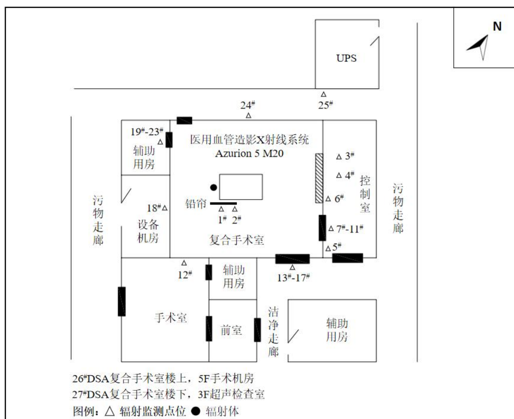
图 6-3 医技楼四楼 DSA 复合手术室辐射环境监测布点示意图
