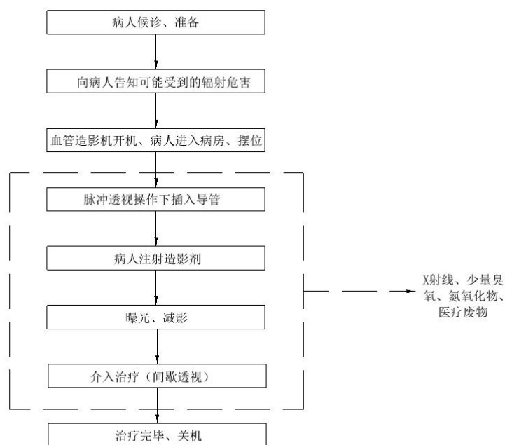
图 2-5 DSA 数字减影介入治疗流程及产污环节示意图
